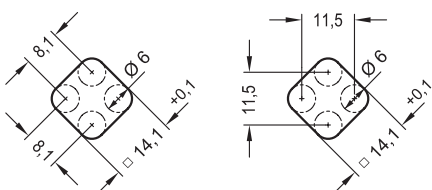
Montagebohrung für Bohren oder Fräsen
