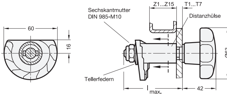
Form SG mit Sterngriff
