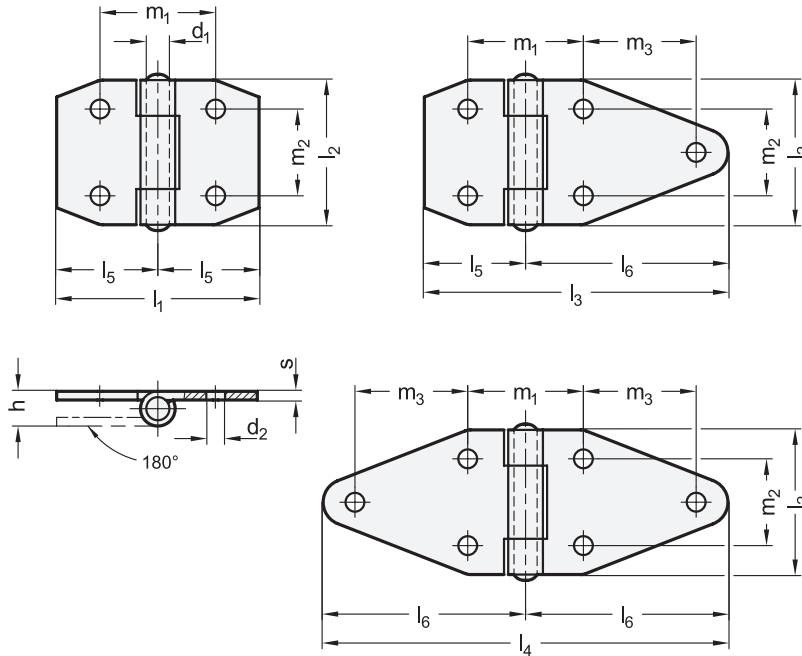
4 Form B mit Durchgangsbohrungen
