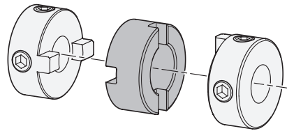
Montagehinweis
