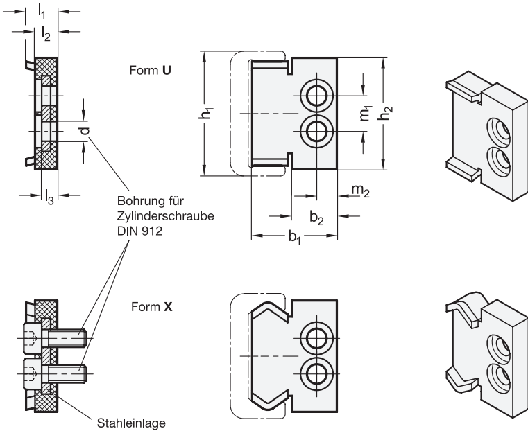
2 Form U für Loslager-Laufschiene X für Festlager-Laufschiene
