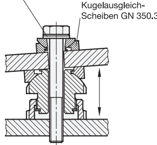
Unterlegscheibe GN 6339
