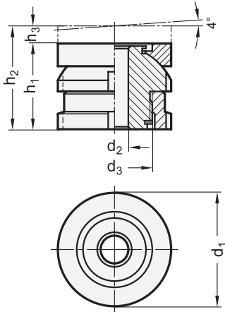
Unterlegscheibe GN 6339
