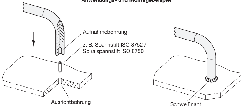
Anwendungs- und Montagebeispiel
