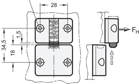
Montagehinweis / Bohrbild
