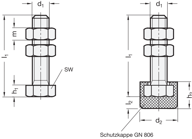
Schutzkappe GN 806
