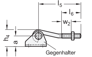
Form TU Zuganker mit Haken
