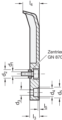
Anbaubeispiel
